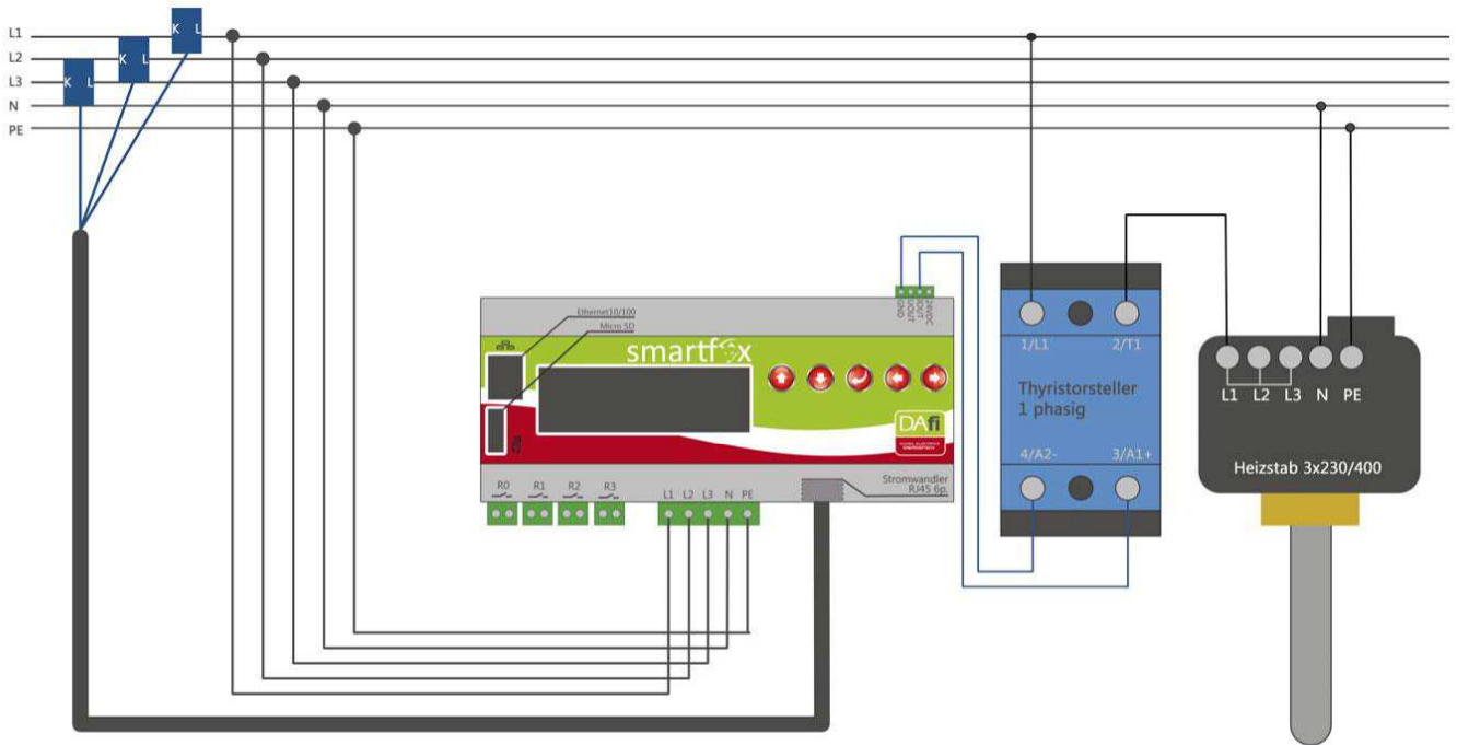
Anschlussbild Thyristorsteller und Heizstab Einphasig
