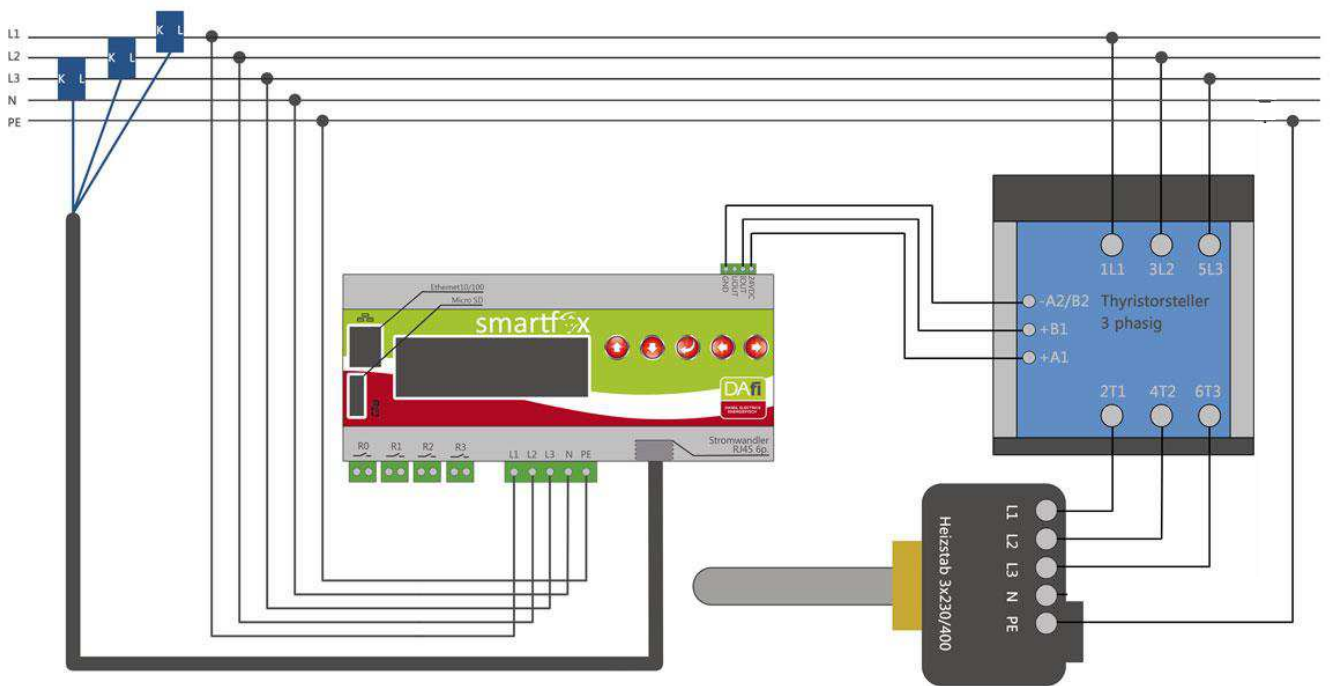
Anschlussbild Thyristorsteller und Heizstab Dreiphasig
